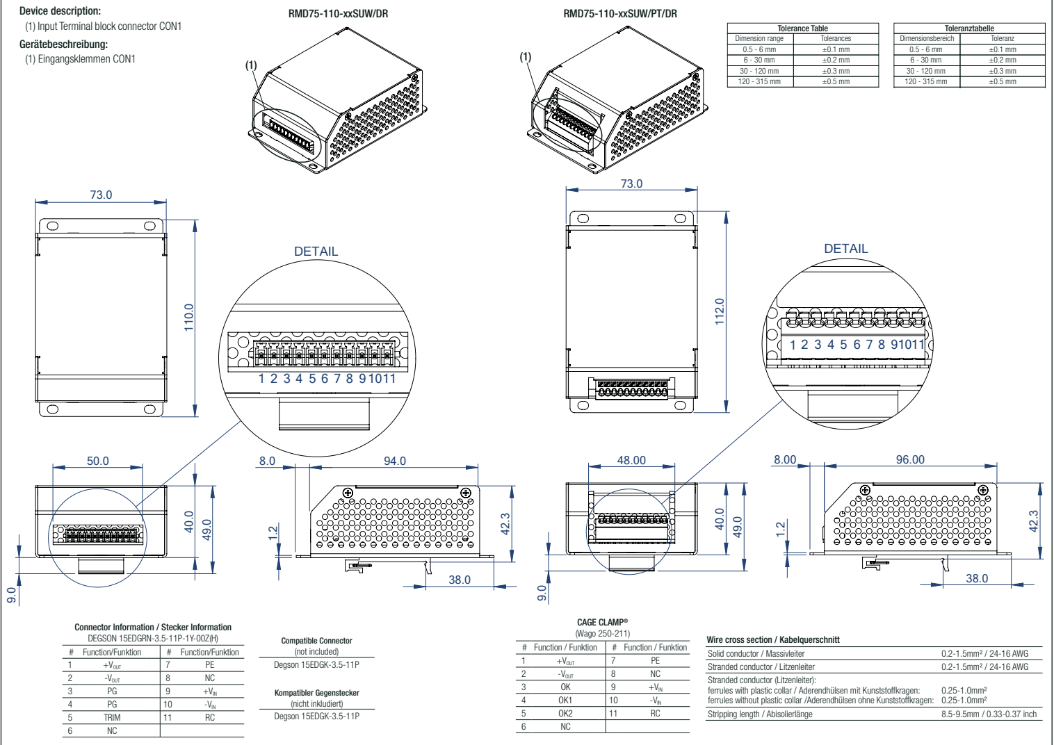
Fig. 2: Mounting Instruction / Abb. 2: Montagerichtlinien
