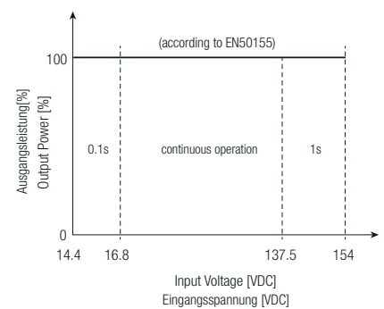
Fig. 4: Input Voltage Range / Abb. 4: Eingangsspannungsbereich
