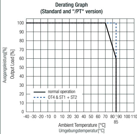
Fig. 3: Derating Graph / Abb. 3: Temperaturverhalten
