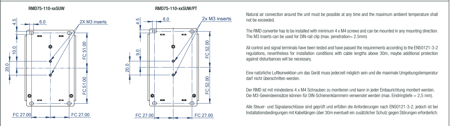
Fig. 2: Mounting Instruction / Abb. 2: Montagerichtlinien
