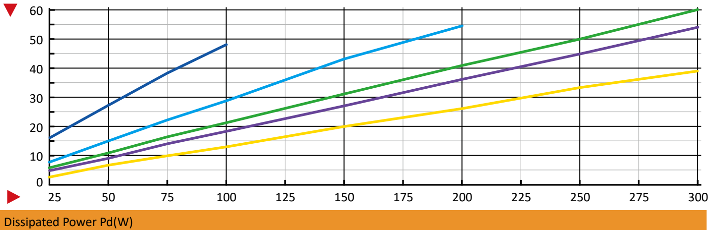
Heat sink to ambient temperature rise T hs-amb (°C)
