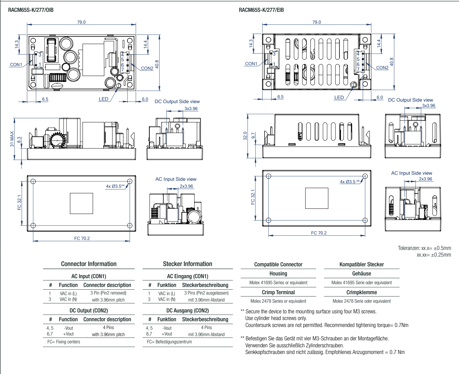
Fig. 1: Mechanical Dimension [mm] / Abb. 1: Mechanische Dimensionen [mm]
