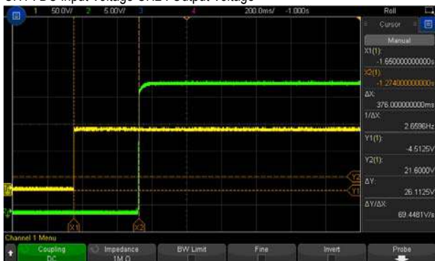
CH1 : DC Input Voltage CH2 : Output Voltage
